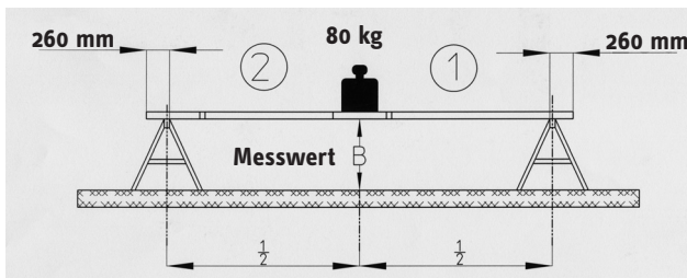
Bild 4: Belastete, umgesteckte Leiterteile mit Prüflast
